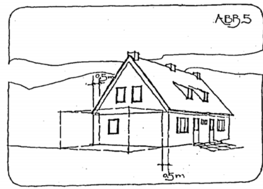
Anbau mit beidseitigem Rücksprung
